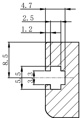
局部C 四面, M3螺母, 安装用 比例: 4: 1
